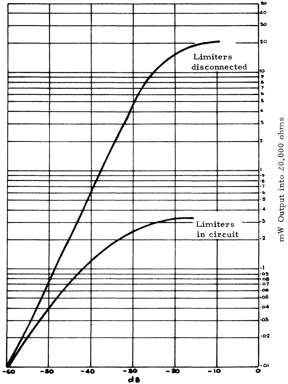
AF Input to TP2: at 1 Kc/s 0db=10 volts
